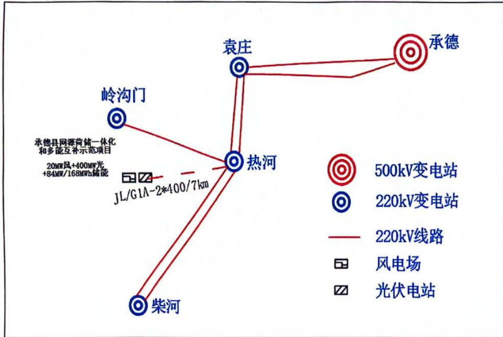
图 2-1 接入系统方案示意图
