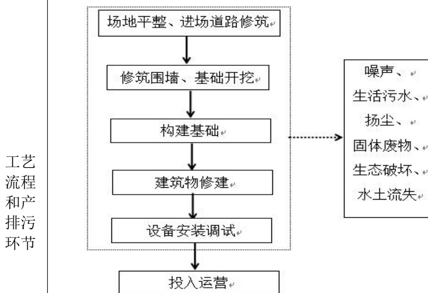
图 2-1 施工期工艺流程及产污节点图
