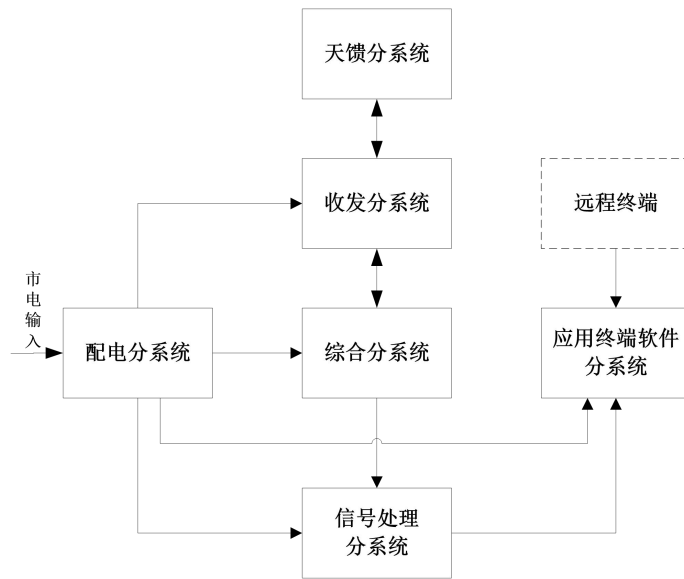
图 2-2 风廓线雷达系统框图
