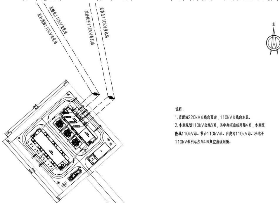
图 2-1 蓝旗变电站出线间隔示意图
