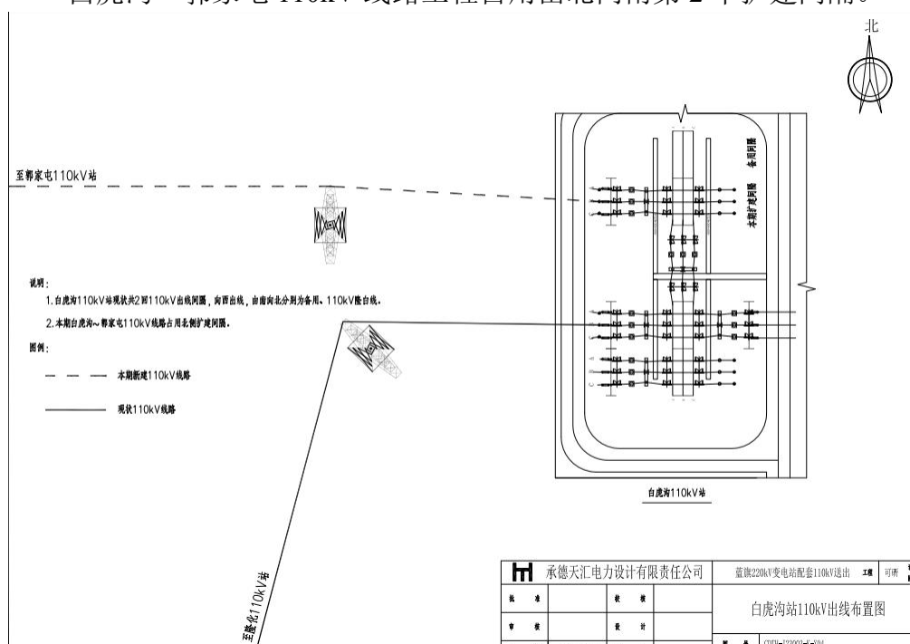
图 2-3 白虎沟变电站出线间隔示意图
