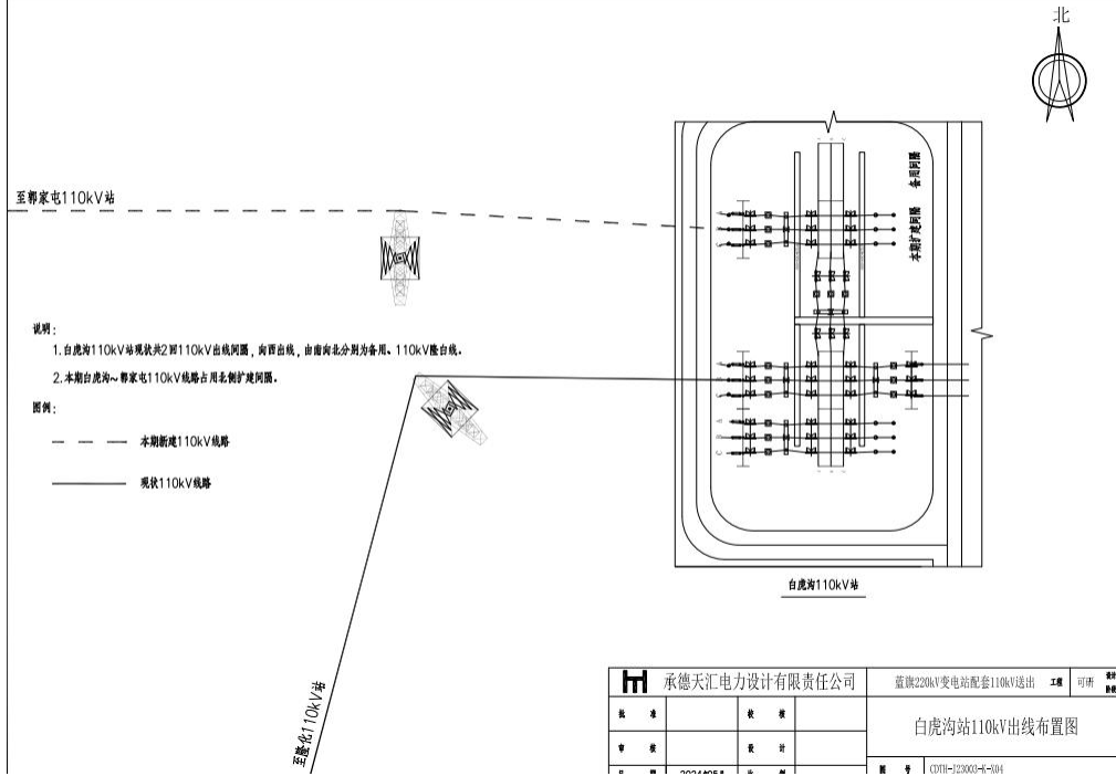
图 2-4 白虎沟变电站出线间隔示意图
