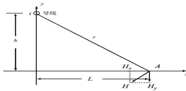
图 5-5 磁场向量图
