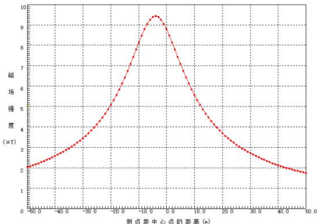
图 5-11 110kV 双回塔单侧挂线线路工频磁感应强度综合量分布曲线图
