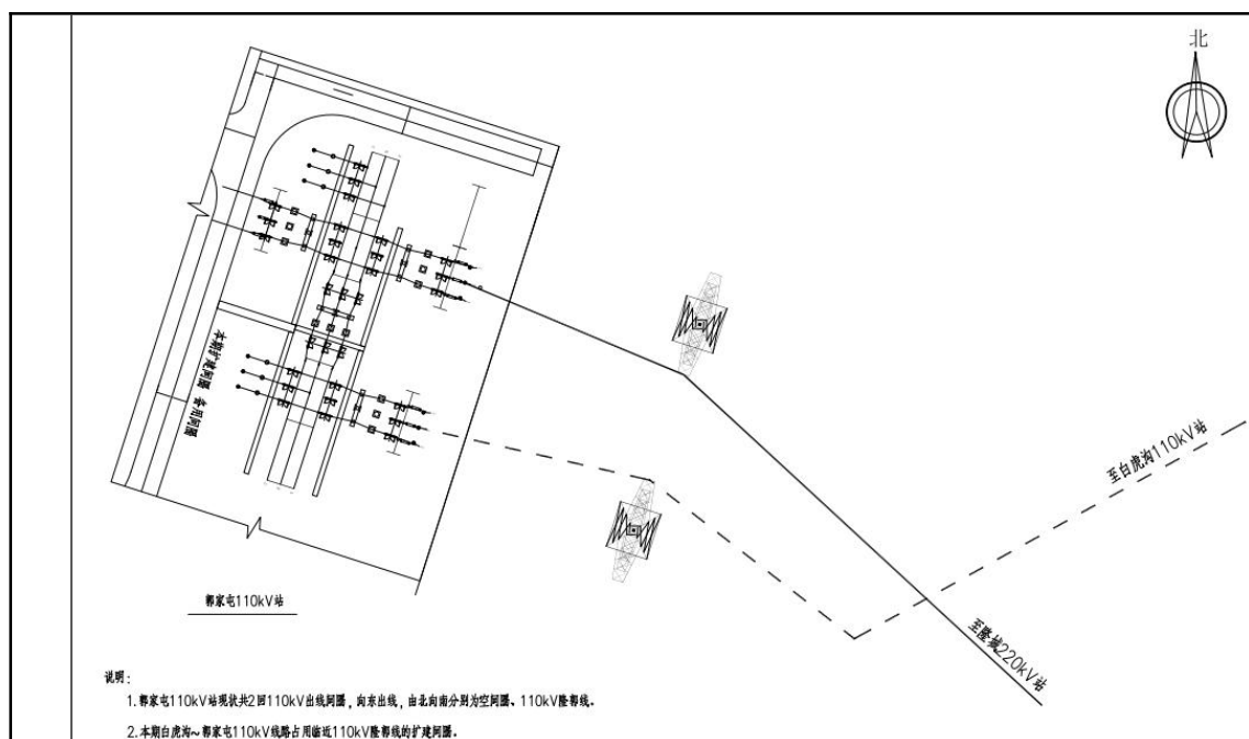
图 2-4 郭家屯变电站出线间隔示意图
