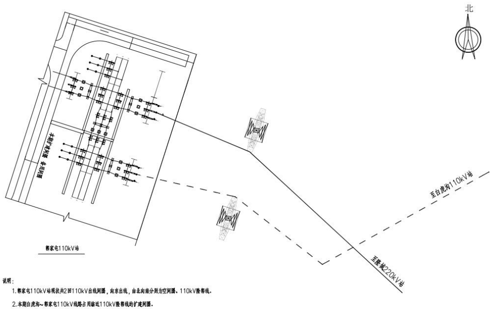
图 2-5 郭家屯变电站出线间隔示意图
