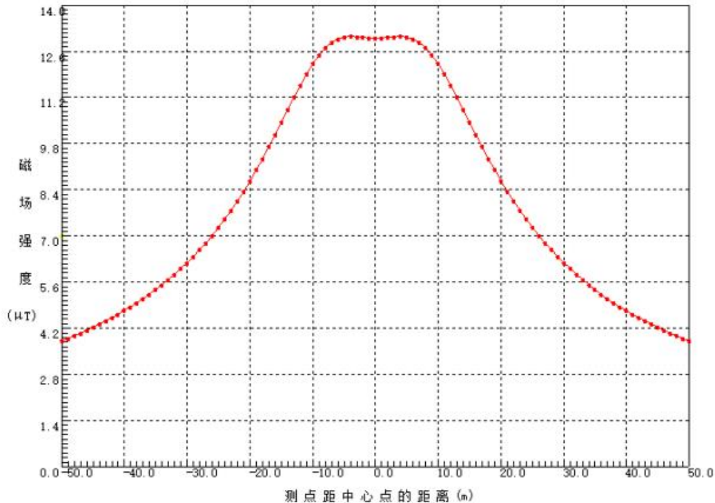
图 5-11 110kV 双回线路工频磁感应强度综合量分布曲线图
