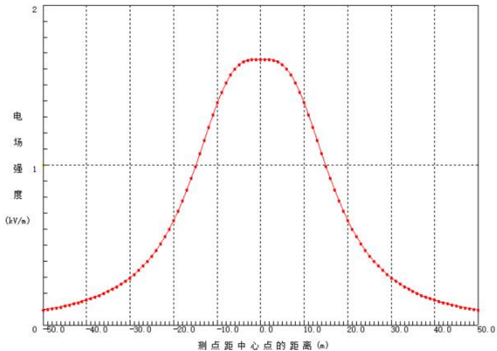
图 5-10 110kV 双回线路工频电场强度综合量分布曲线图
