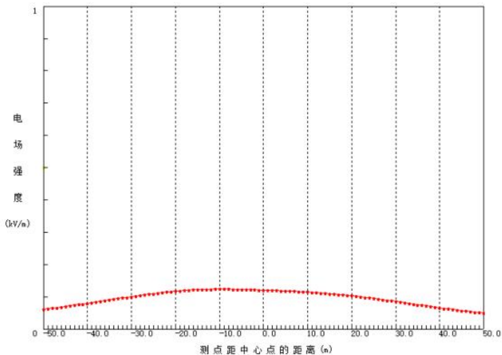
图 5-7 110kV 单回线路工频电场强度综合量分布曲线图
