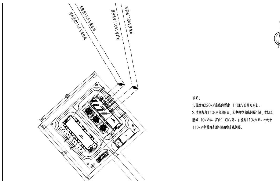
图 2-1 蓝旗变电站出线间隔示意图
