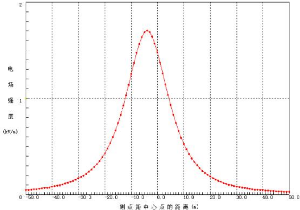
图 5-10 110kV 双回塔单侧挂线线路工频电场强度综合量分布曲线图
