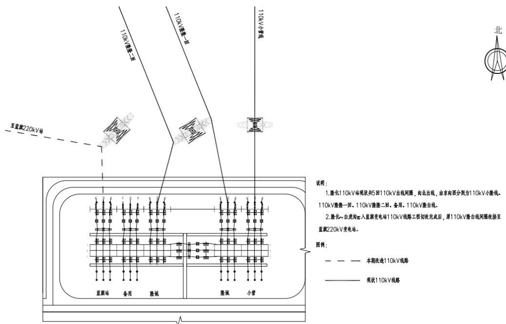
图 2-2 隆化变电站出线间隔示意图
