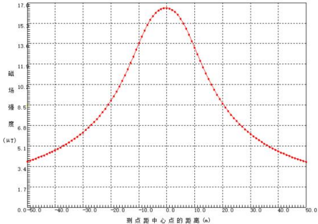
图 5-8 110kV 单回线路工频磁感应强度综合量分布曲线图
