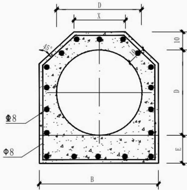
360° 基座断面 (D≤1000)
