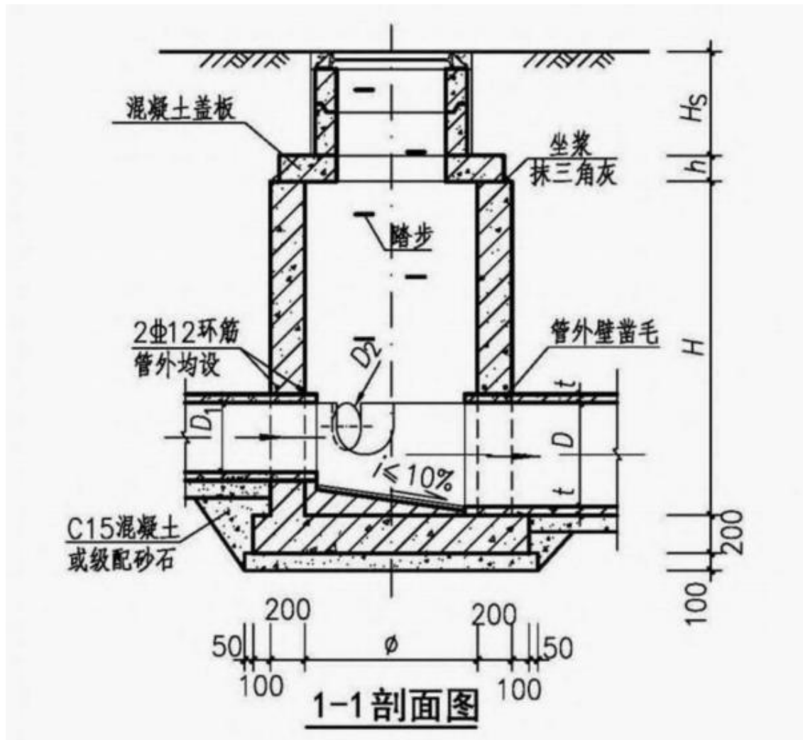
图 2-4 项目污水井及管道接口剖面图
