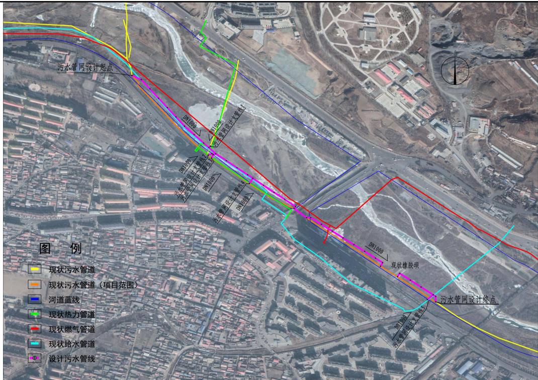
图 2-1 河道现状管线总平面图
