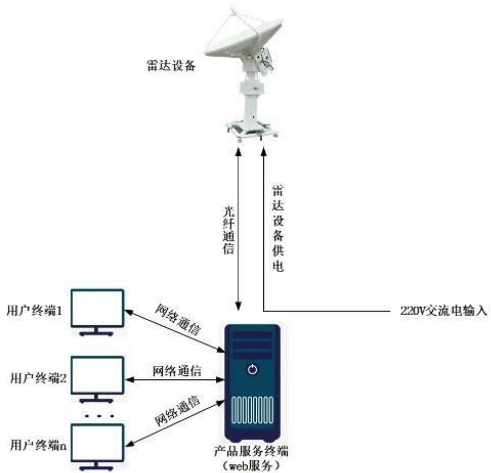
图 2.2 硬件结构示意图
