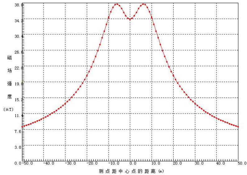
图7 单回路塔 220kV 架空线路路段磁感应强度分布图
