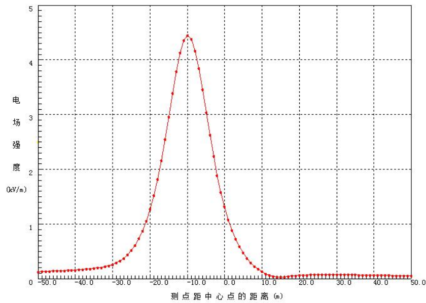
图 6 双回路塔单侧挂线 220kV 架空线路路段电场强度分布
