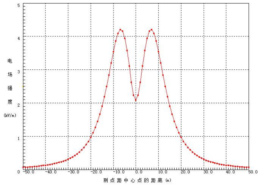
图 5 单回路塔 220kV 架空线路路段电场强度分布
