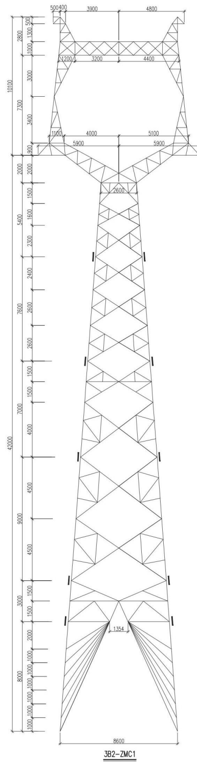
图 1-1 预测塔型图
