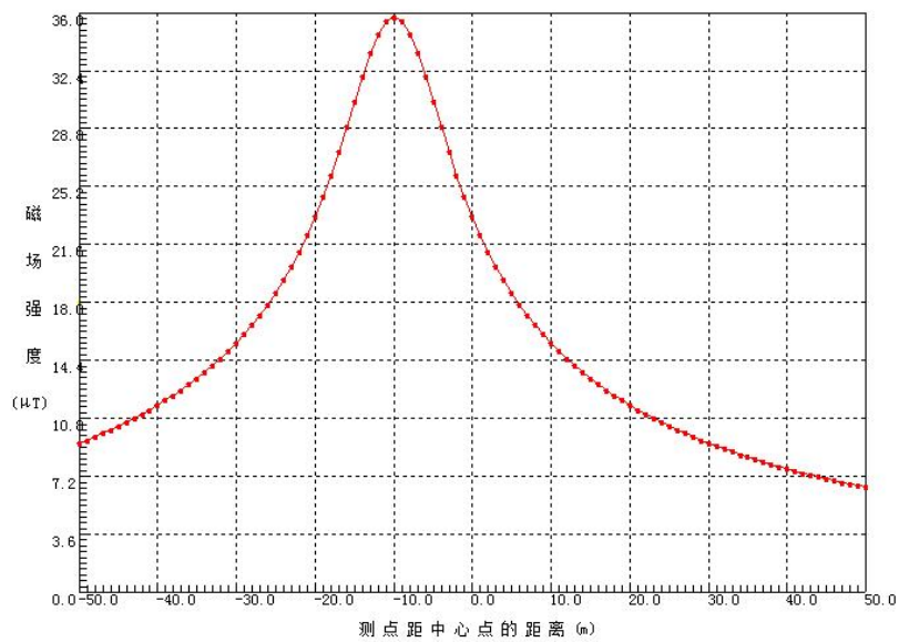
图8 双回路塔单侧挂线 220kV 架空线路路磁感应强度分布图
