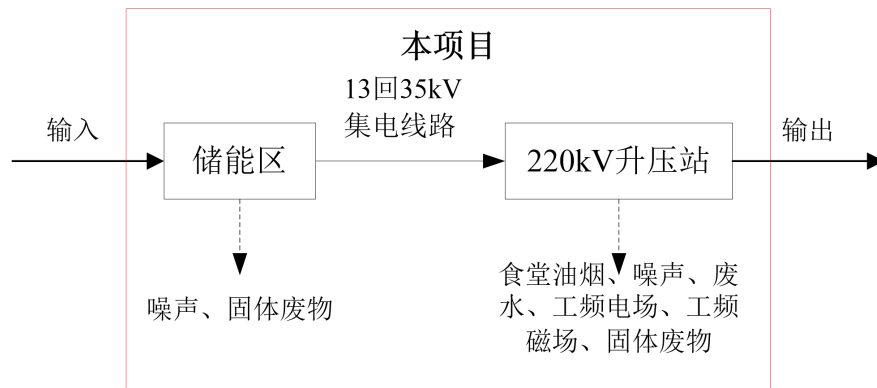
图 2-2 工艺及产污节点图
