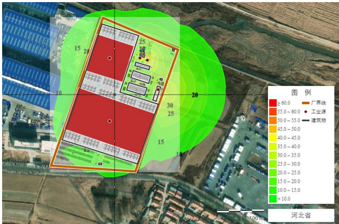
图 4-1 预测结果等声级线值
